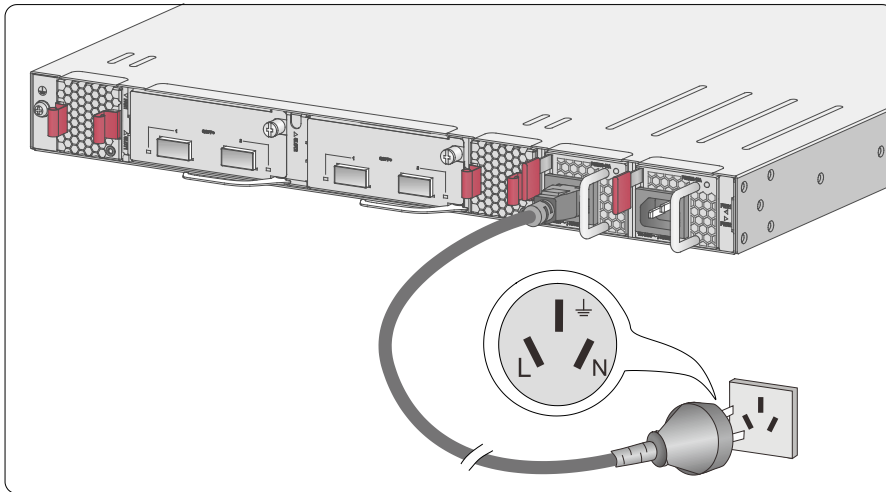
图2-18 利用交流 PE 线接地时接地安装示意图
