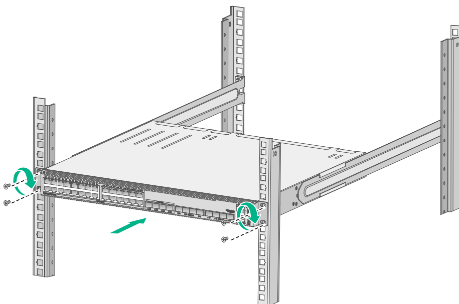
图2-15 安装交换机到机柜示意图（挂耳安装在靠近端口侧）
