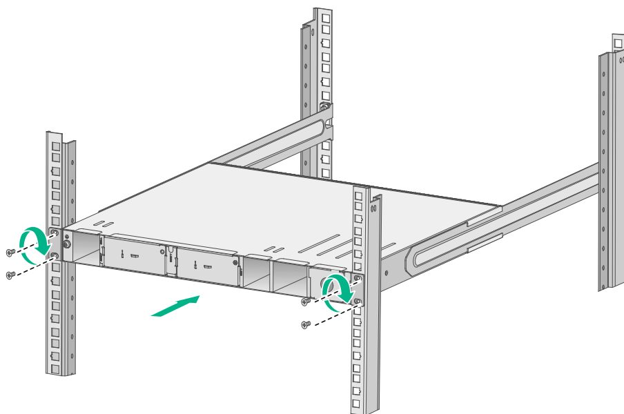
图2-14 安装交换机到机柜示意图（挂耳安装在靠近电源侧）
