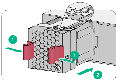
图2-19 风扇模块安装示意图
