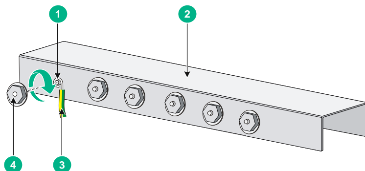
图2-17 连接接地线缆到接地排
