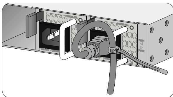
图2-26 交流电源线连接示意图
