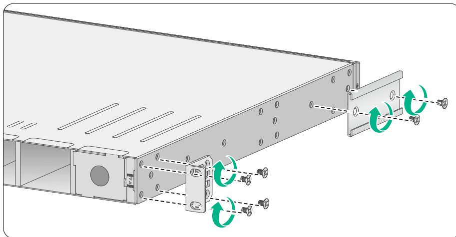
图2-12 安装挂耳和滑道导轨到机箱的示意图（以长滑道导轨为例）
