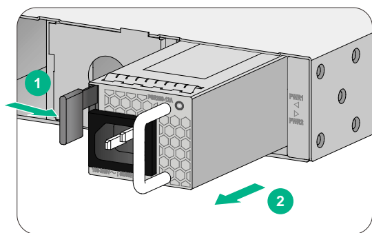
图2-25 拆卸电源模块示意图
