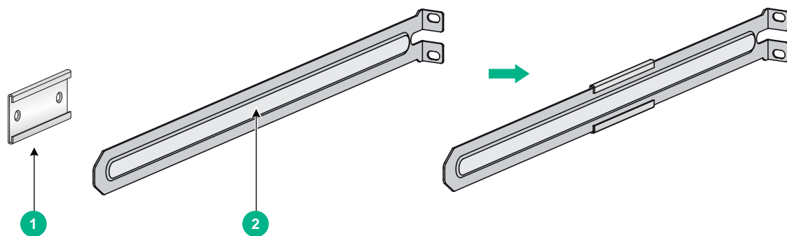
图2-6 1U 滑道及滑道导轨示意图（以长滑道为例）
