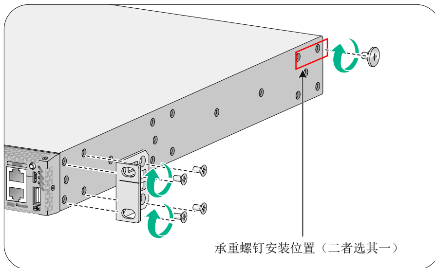
图2-7 安装前挂耳和承重螺钉到设备的示意图
