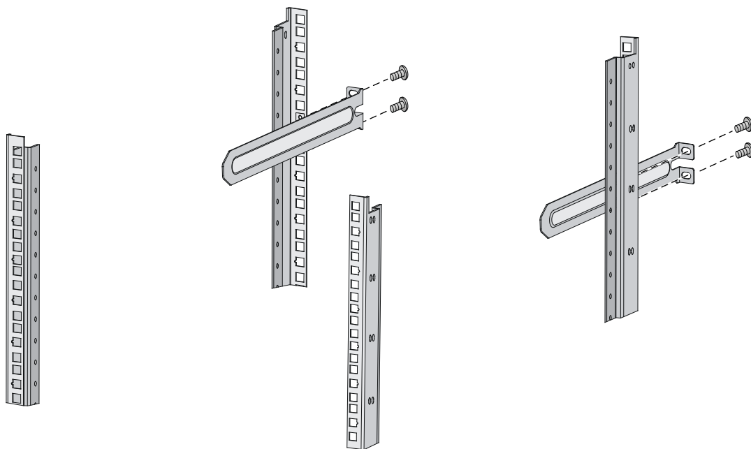
图2-13 滑道安装示意图（以长滑道为例）
