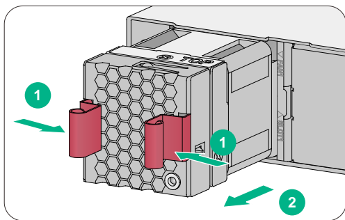
图2-20 风扇模块拆卸示意图
