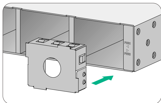
图2-24 电源假面板安装示意图
