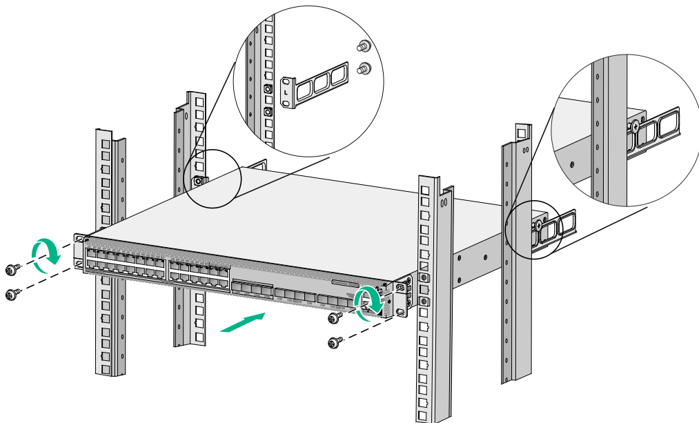
图2-11 安装交换机到机柜示意图（后挂耳反向安装到机柜方孔条）
