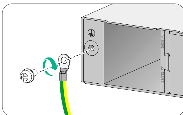
图2-16 连接保护地接线到交换机的接地孔
